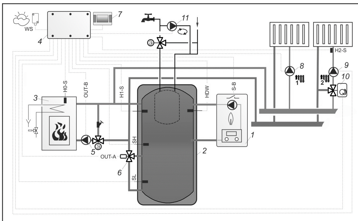
Рис. 25 Схема с тепловым буфером с послойным нагревом буфера 7 , где: 1 – котел, 2 – тепловой буфер, 3 – камин с водяным контуром, 4 – силовой модуль, 5 – насос камина с водяным контуром, 6 – переключающий клапан, 7 – панель управления с функцией комнатного термостата, 8 – насос нерегулируемого отопительного контура H1, 9 – насос смесительного контура H2, 10 – сервопривод смесительного клапана контура H2, 11 - циркуляционный насос ГВС, H1-S – датчик верхней температуры буфера тип СТ4, SH – датчик средней температуры буфера тип СТ6, SL – датчик нижней температуры буфера тип СТ6-W, WS - датчик наружной температуры СТ6-P, датчик температуры бойлера ГВС.
